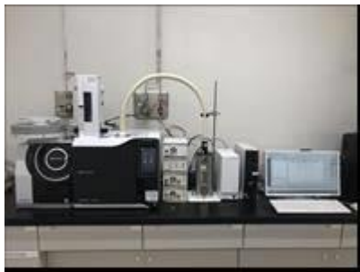
図1 フタル酸エステル類等スクリーニング装置
