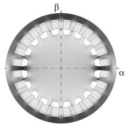
図2 固定子および回転子の形状
