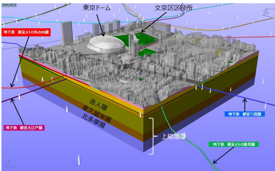
図－1 文京区における3次元地質モデルと地下施設モデルの合成
